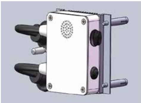
Figur 1: Installieren Sie zunächst IHBD3 an die Wand.
