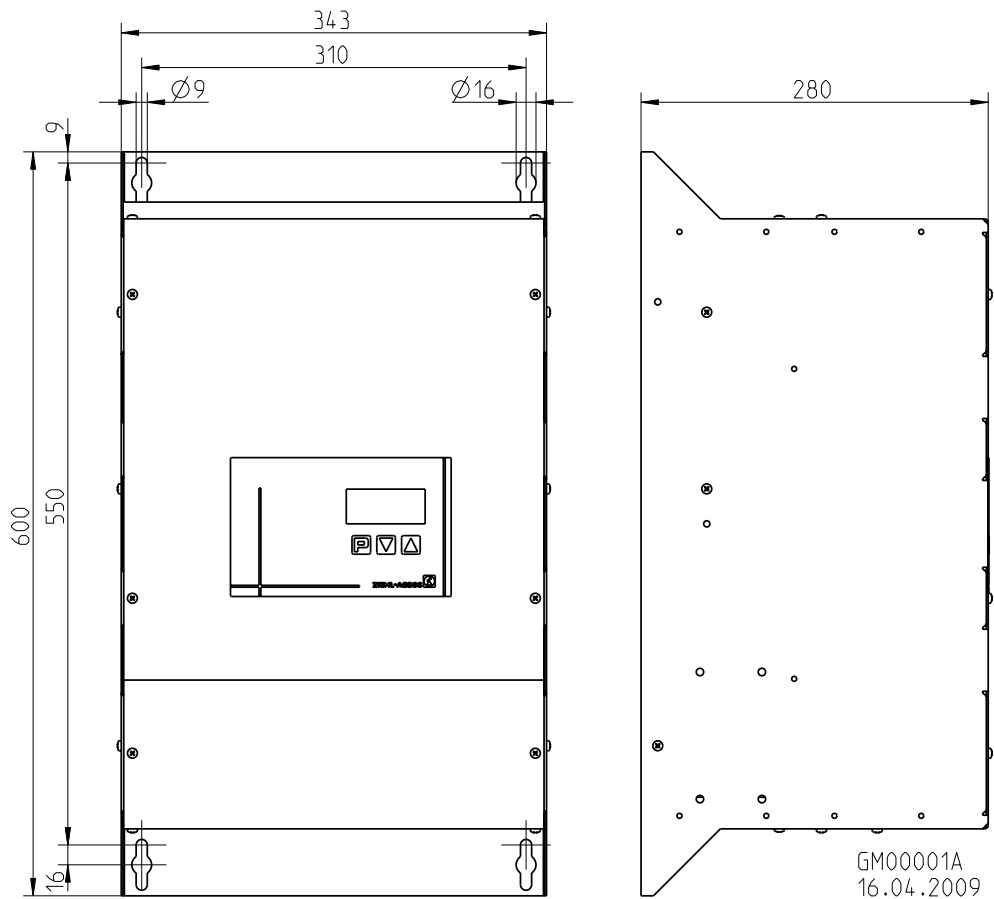
FXDM32...50E (IP20)
