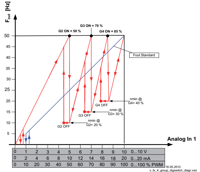
Beispiel: Zuschaltung von 3 Gruppen über Relais
