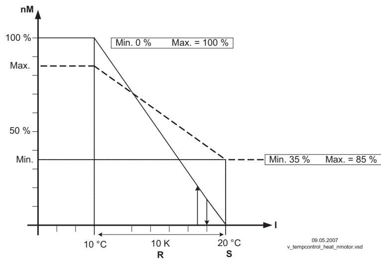
Beispiel 2: Temperaturregelung in “Heizfunktion” (idealisiertes Prinzipschaubild)
