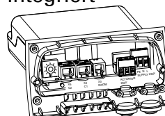
SIReB1, integrierte Basisleiterplatte
