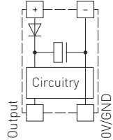
Schéma de raccordement individuel
