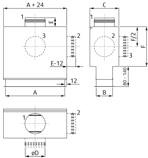
Fig. 15: The ODEN plenum box basic dimensions
