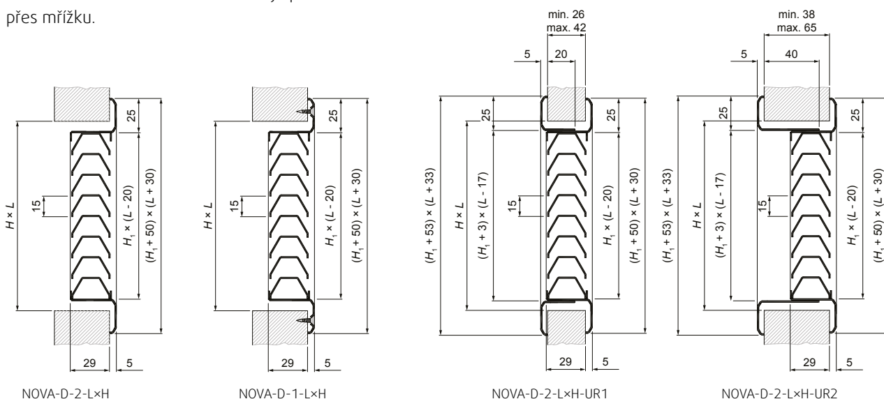
Obr.1: Rozměry mřížek
