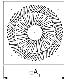
VVKR-A-S-800-72
