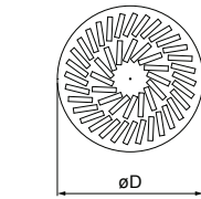
øD VVKR-A-R-600-48 625
