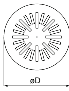
øD VVKR-B-R-500-24 600 625
