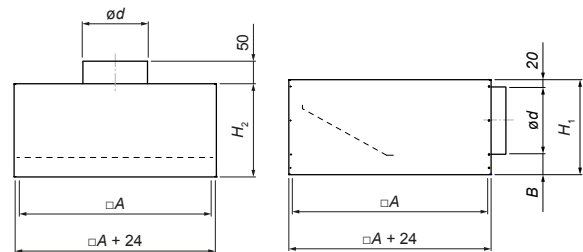
Obr. 7: Rozměry pro čtvercové plenum boxy PB-VVK-S
