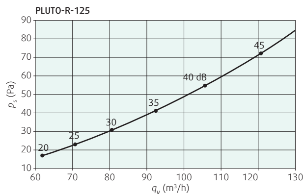
Graf 1: Tlaková ztráta a hladina akustického výkonu L_{W(A)}
