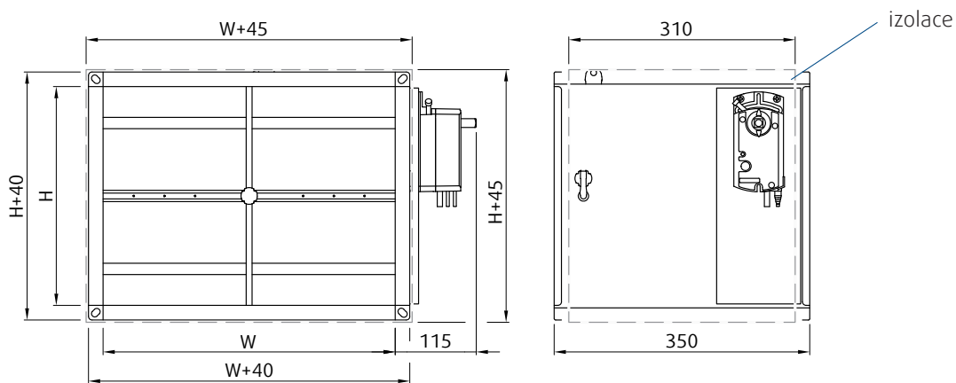
Obr. 4: Rozměry OPTIMA-S a OPTIMA-SI při H = 100, 200 \dots 1000 mm
