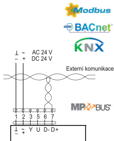
Obr. 8: Schéma zapojení pro externí komunikaci
