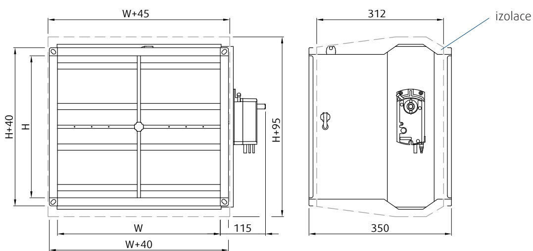
Obr. 5: Rozměry OPTIMA-S a OPTIMA-SI při H = 150, 250 \dots 950 mm
