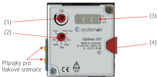
Obr. 9: Ovládací panel servopohonu GO-MOD
