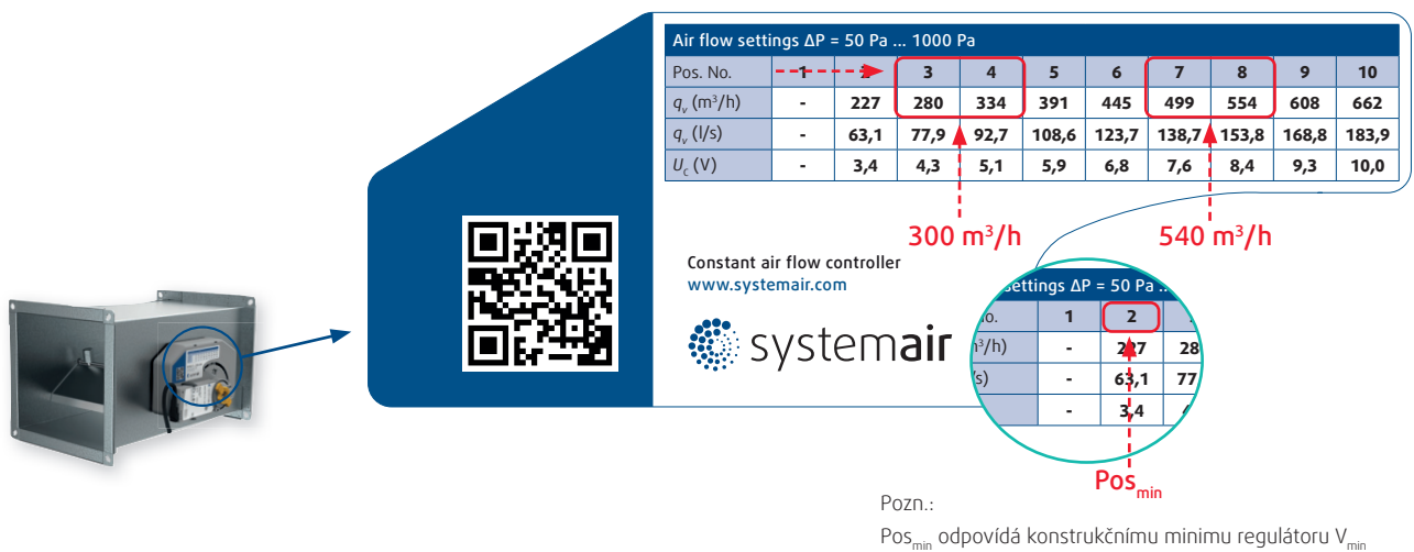
Obr. 9: Detail štítku regulátoru NOTUS-S-M1 pro nastavení průtoku vzduchu
