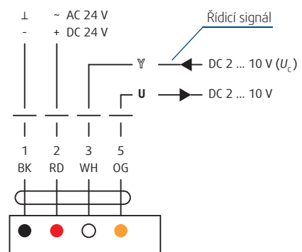
El. schéma 2
