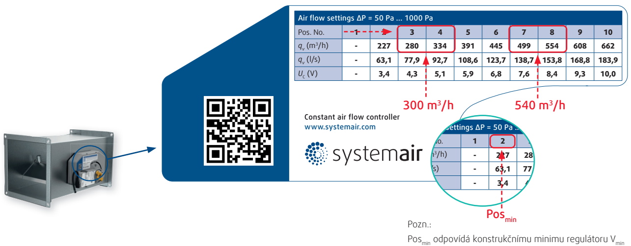
Obr. 10: Detail štítku regulátoru NOTUS-S-M2 pro nastavení průtoku vzduchu
