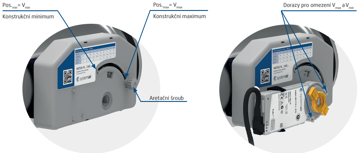
Obr. 2: Detail mechanismu pro nastavení průtoku vzduchu
