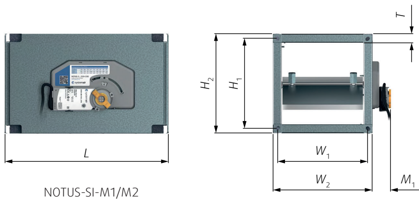
Obr. 5: Rozměry NOTUS-S a NOTUS-SI
