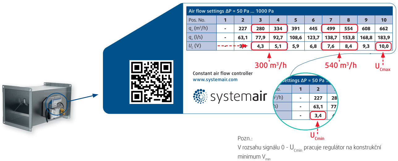
Obr. 8: Detail štítku regulátoru NOTUS-S-M1 pro nastavení průtoku vzduchu
