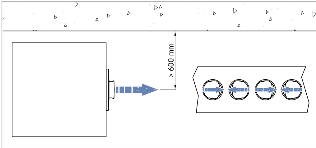
Messanordnung
